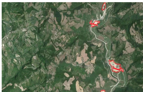
Figura 76 - Primo lotto della diga di Casanuova per sbarrare lo scorrimento del fiume Chiascio, allo scopo di creare, entro la fine del 2019, un serbatoio idrico per l'utilizzo agricolo. L'area si trova nel territorio di Gubbio, a confine tra il suo perimetro urbano e quello del contermino Comune di Valfabbrica (PG). Inoltre, nell'area più a valle, sono stati eseguiti importanti lavori di sterro all'interno dell'alveo fluviale.
