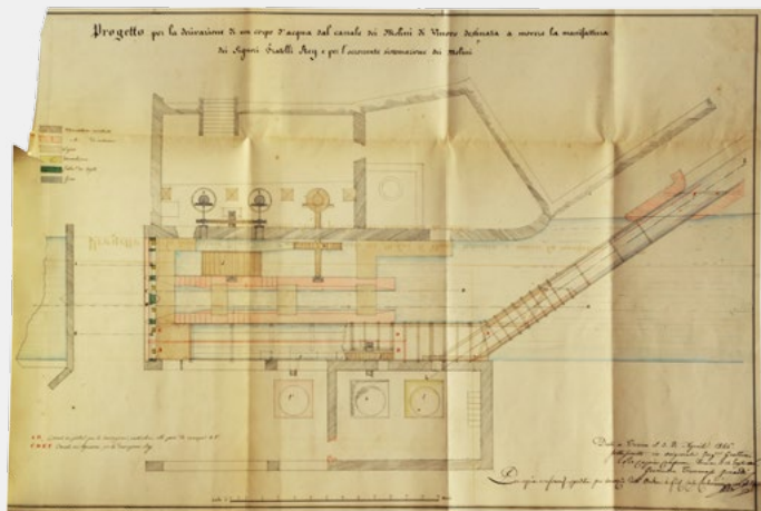
Ing. GRATTONI, Progetto per la derivazione di un corpo d'acqua dal canale dei Molini di Vinore destinata a muovere la manifattura dei Signori Fratelli Rey e per l'occorrente sistemazione dei Molini , 1846. AOM, Custodia degli Instrumenti 1846 (8), c. 24, 1846.
