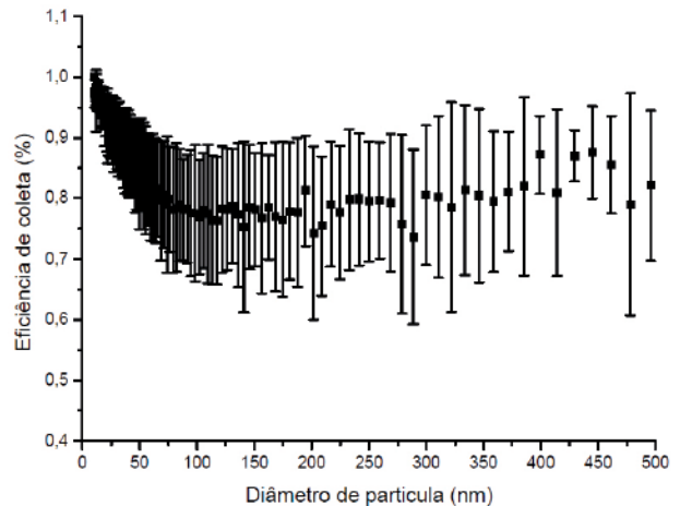
Figura 7: Média de eficiência de coleta do filtro de nanofibra 2
