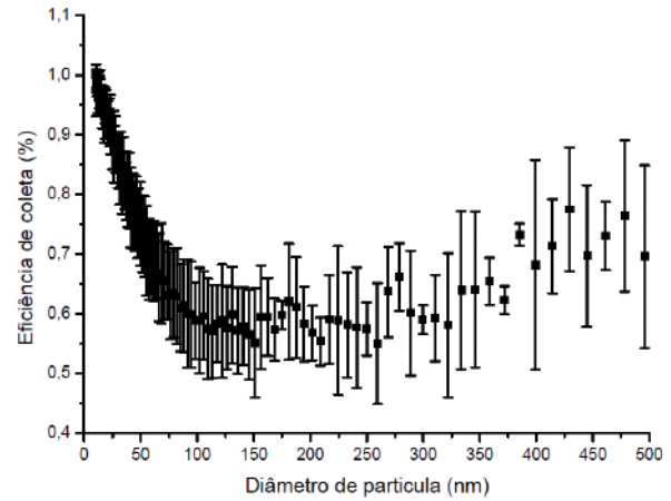
Figura 6: Média de eficiência de coleta do filtro de nanofibra 1
