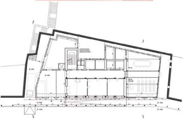
[Fig. 29 - ex scuola di Sampeyre - schemi esemplificativi delle possibilità di sfruttamento e di ampliamento totali - DICAS]
