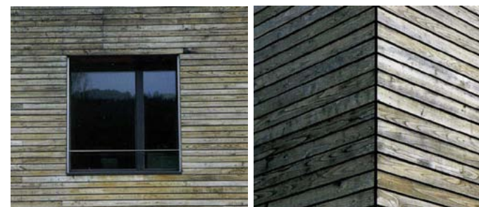
[Fig. 9-10 - dettaglio di involucro di residenza per studenti a Wuppertal - progettisti: fase 1 - PPP con Michael Muller e Christian Schluter, Dusseldorf; fase2 - architektur contor Muller Schluter, Wuppertal]
