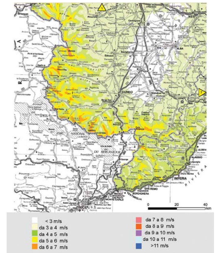
[Fig. 10 - cuneese - velocità media annua del vento a 50 m s.l.t. - mappa elaborata da CESI in collaborazione con il dipartimento di Fisica dell'Università di Genova nell'ambito della ricerca di Sistema - fonte: GEONEX, De Agostini, 2002 - atlante eolico italiano - velocità media annua del vento a 50 m s.l.t./s.l.m.]
