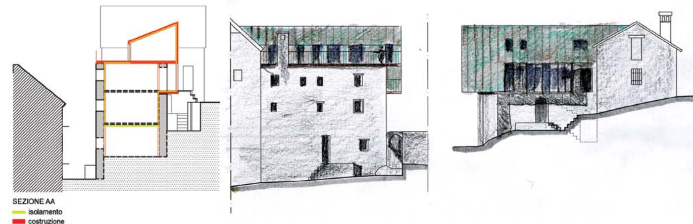
[Fig. 25 - aumento di cubatura: intervento senza mimetismi, mantenimento delle caratteristiche della preesistenza nel rispetto dei vincoli esistenti. A sinistra: sezione. Al centro e a destra: prospetto sud- ovest, e nord est - scala 1:200]
