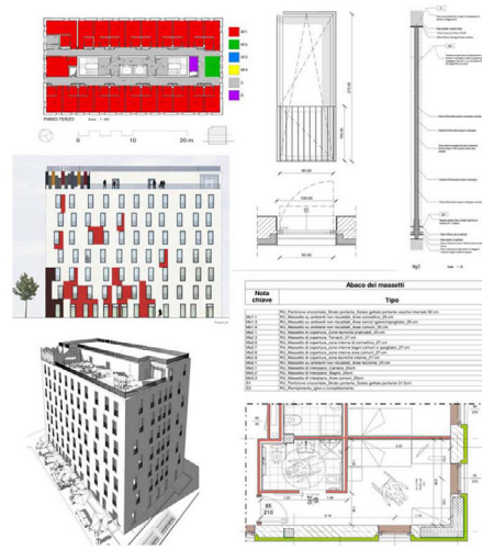
Progettazione architettonica esecutiva della Residenza C. Codegone. Partecipazione al bando ministeriale per l'attribuzione di finanziamenti. Importo lavori circa 11mln €. Committente Politecnico di Torino - 2011
