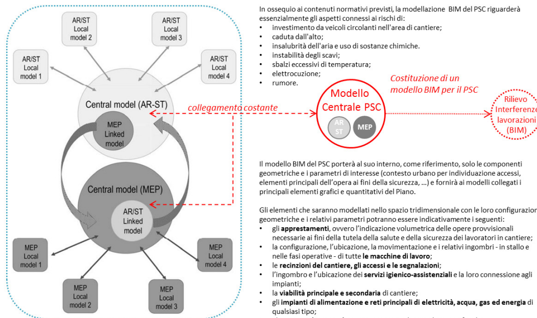
Possibile organizzazione del gruppo di progettazione in ambiente BIM (con modelli collegati o con workset)
