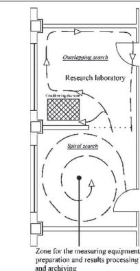
Fig. 9. Layout of the Lab. Planimetria del laboratorio.
