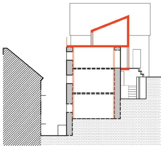
SEZIONE AA
