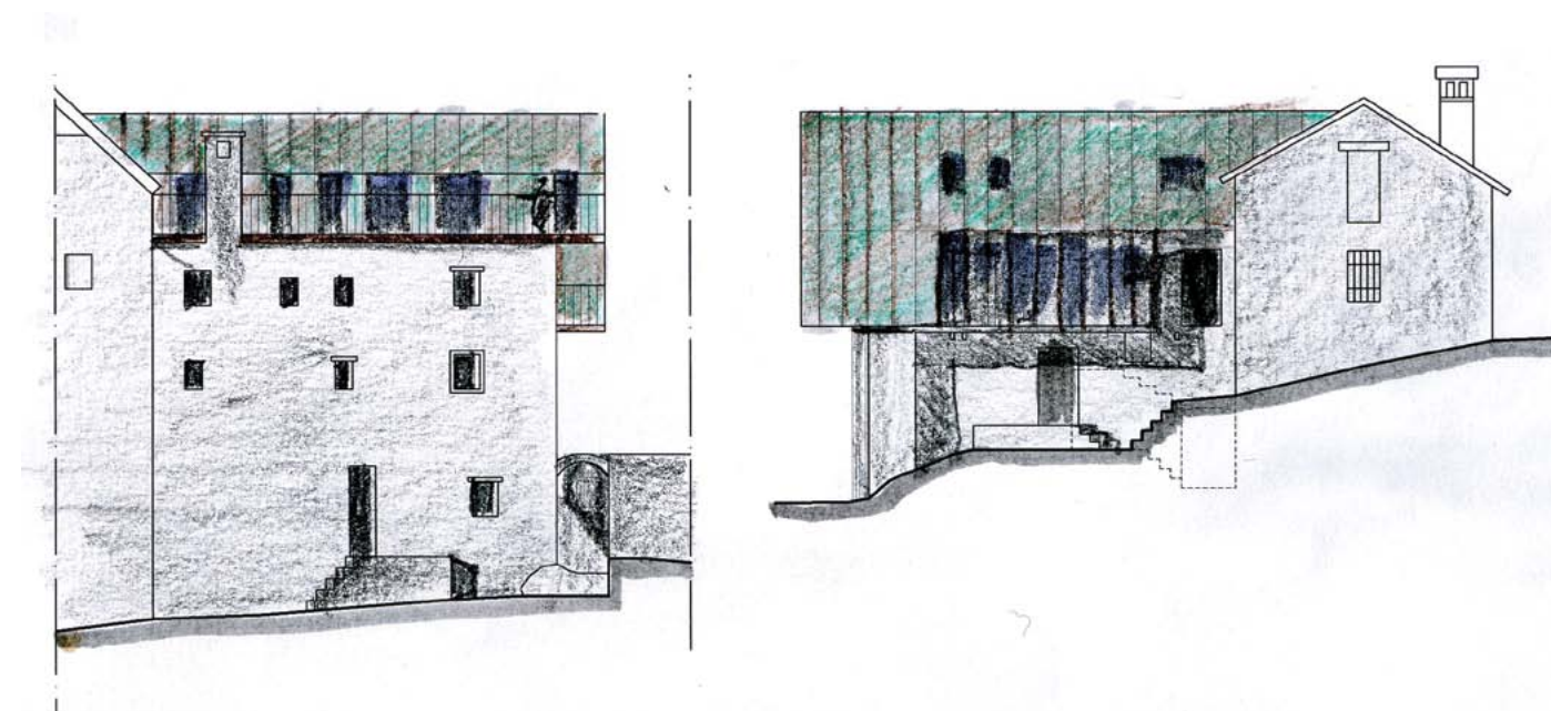
[Fig. 20 - prospetto sud-ovest, e nord est - scala 1:200]
