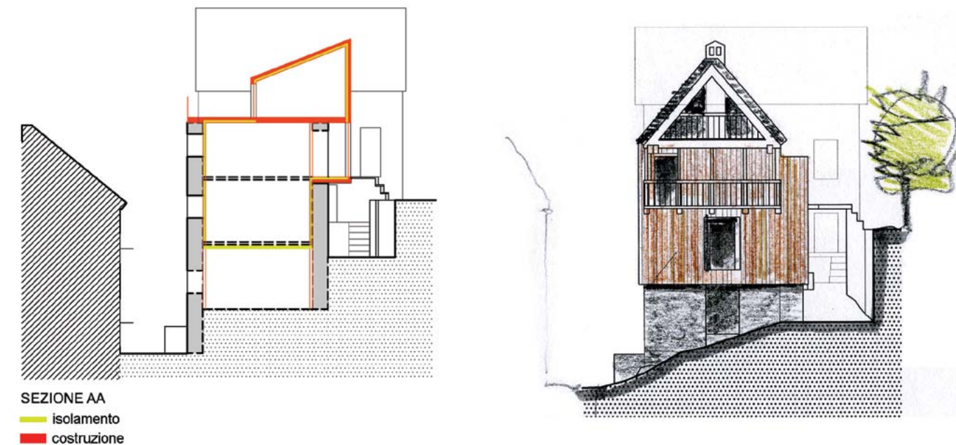
[Fig. 21 - Aumento di cubatura: intervento senza mimetismi, mantenimento delle caratteristiche della preesistenza nel rispetto dei vincoli esistenti - scala 1:200]
