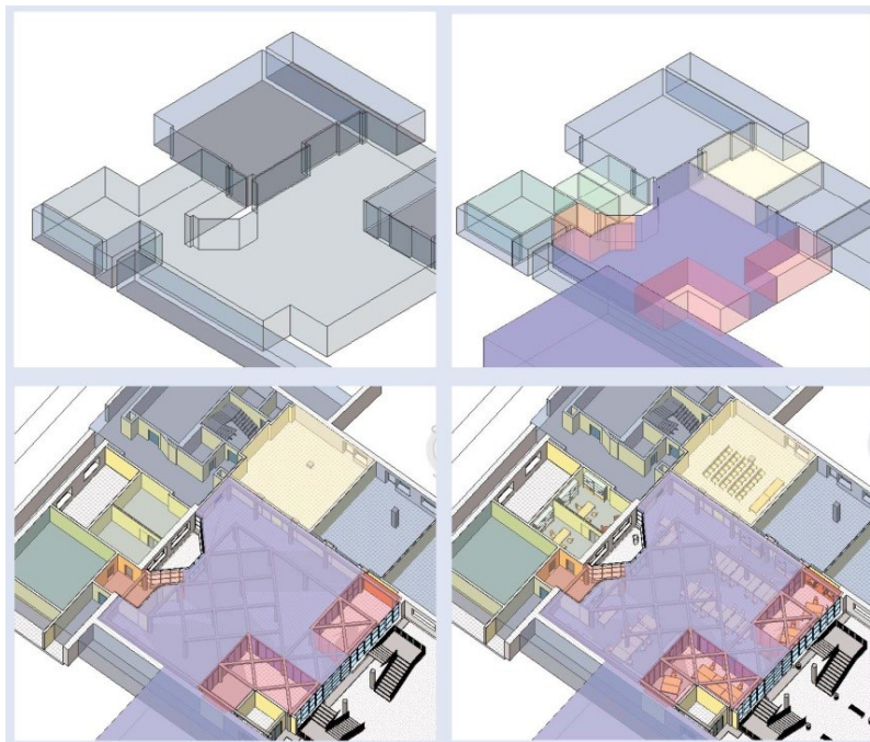
Figura 1 Rappresentazione spaziale dell'intervento relativo al nuovo Centro Linguistico di Ateneo (CLA) secondo quanto richiesto all'interno della Senate Properties BIM's requirement . Il patrimonio infografico è crescente in senso orario. Elaborazione a cura dell'ing. M. Vozzola
