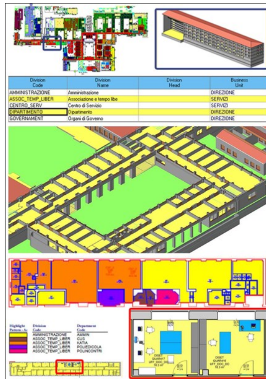
Figura 2 Le diverse visualizzazioni di un modello parametrico utilizzato per operazioni di Facility Management . Elaborazione a cura dell'ing. D. Dalmasso
