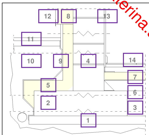
Figura C.1. indicazioni di posa
