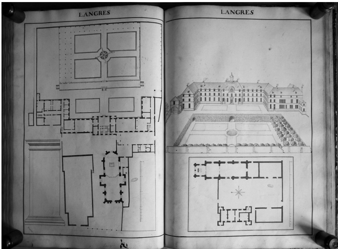
30. Disegnatore ignoto, Pianta e alzato del seminario di Langres e del priorato di Grossauve, penna e inchiostro bruno, su preparazione a matita, acquerellato in grigio, verde e rosso, 1690-1710 circa. Parigi, Archives nationales, Cartes et plans , N IV Seine 68, foll. 44-45.
