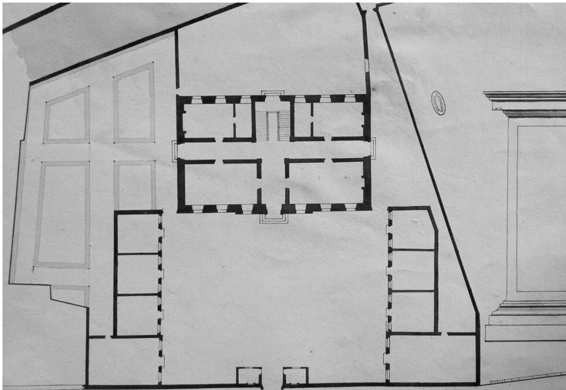
21. Disegnatore ignoto, Pianta del collegio dell'Oratorio di Beaune, penna e inchiostro bruno, su preparazione a matita, acquerellato in grigio e verde, 1690-1710 circa.
