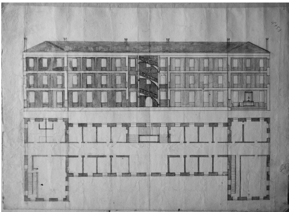
25. Disegnatore ignoto, Progetto per il nuovo seminario di Vienne; pianta su due livelli, prospetto e sezione trasversale. Penna e inchiostro bruno, su preparazione a matita, acquerellato in grigio, 1682 circa. Archives Nationales, Cartes et plans, N IV Seine 69, fol. 31 (recto e verso).
