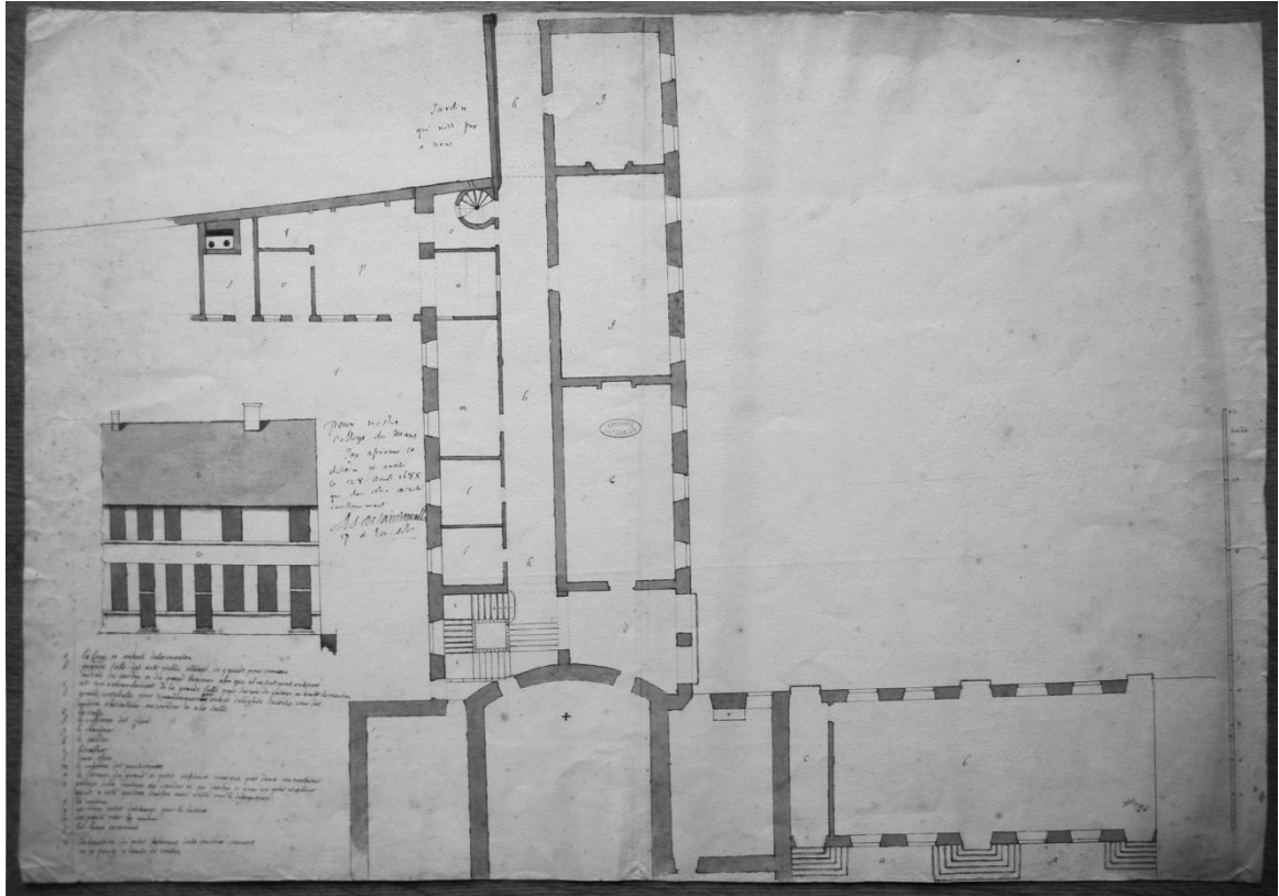
1. Disegnatore ignoto, Progetto per la manica nuova del collegio dell'Oratorio di Le Mans, penna e inchiostro bruno, su preparazione a matita, acquerellato in grigio con velature in bistro, 1688. Parigi, Archives nationales, Cartes et plans , N III Sarthe 3/2.
