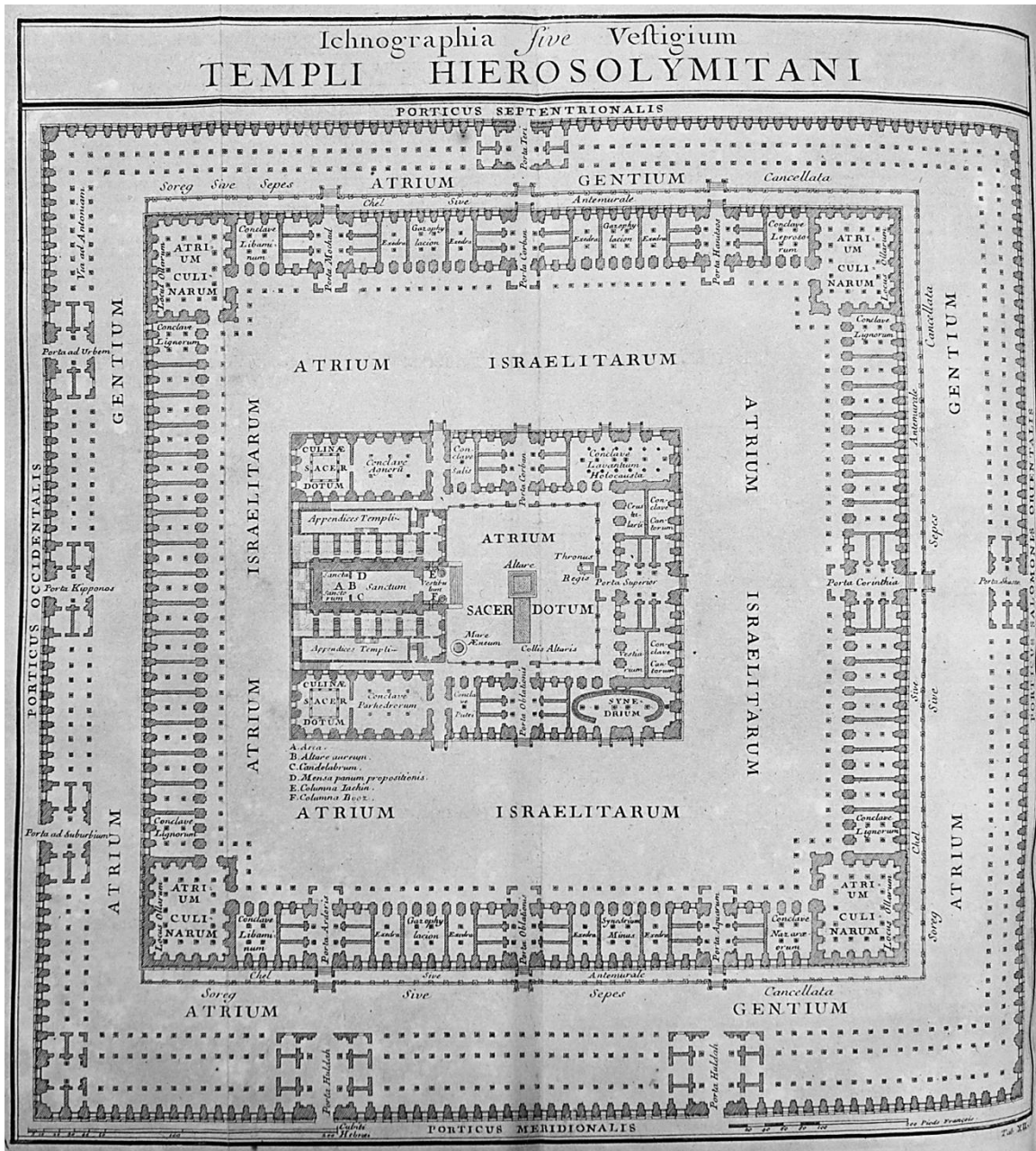
13. [F. Delamonce] (su disegno di), Pianta del Tempio di Gerusalemme nella versione definitiva, bulino. La pianta è ricalcata sulla seconda restituzione, ma ruotata di 90°. Da B. Lamy, De Tabernaculo Fœderis... , D. Mariette, Paris 1720, tav. XII.
