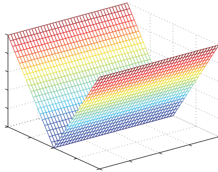
FIG. 3.2. Function \Psi(\hat{x}) .
