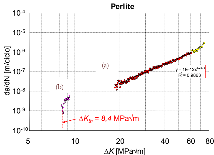
Figura 4: Determinazione sperimentale di curve di propagazione per fatica di cricca per una struttura perlitica (a) e del relativo valore di \Delta K di soglia, \Delta K_{th} (b) ( R=0,1 ).
