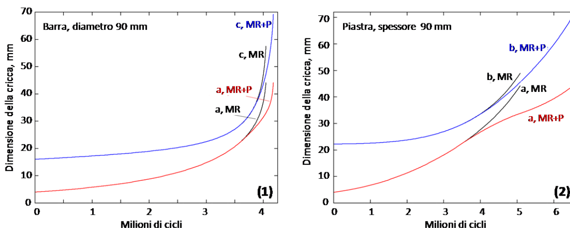
Figura 15: Calcolo della crescita per fatica della profondità (a) e dalla semi-larghezza circonferenziale (c) di una cricca in una barra cilindrica di 90 mm di diametro con martensite rinvenuta (MR) in tutta la sezione o con perlite a cuore (MR+P) (1) o della crescita della cricca in profondità (a) ed in semi-larghezza (b) in una piastra di 90 mm di spessore con gli stessi costituenti metallografici (2).
