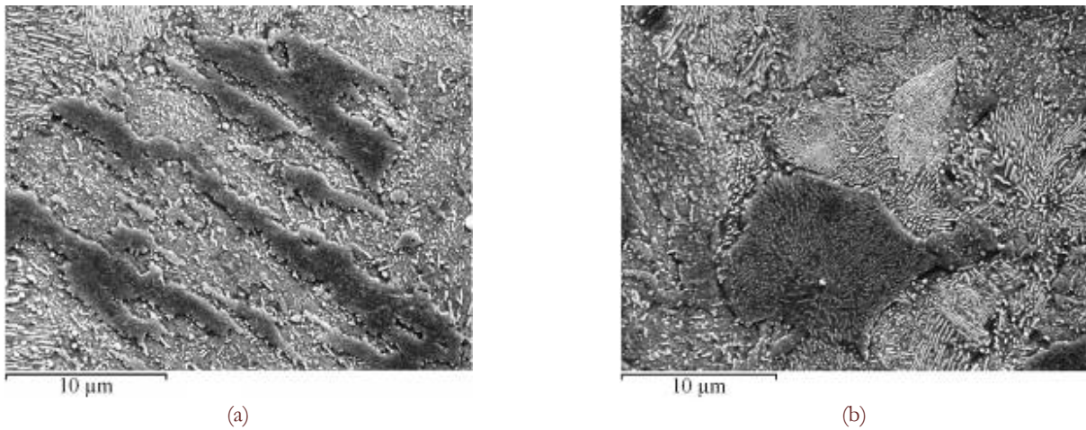
Figura 3: Microscopia elettronica a scansione dei costituenti metallografici di Fig. 2d: bainite superiore modificata dal rinvenimento (a) e perlite fine (b). Attacco Nital.
