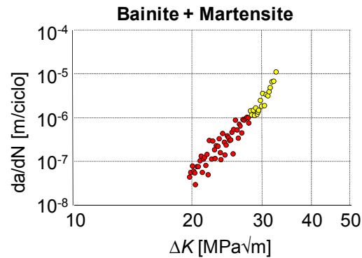
Figura 6: Determinazione sperimentale di curve di Paris per una struttura mista bainitico-martensitica ( R=0,1 ).
