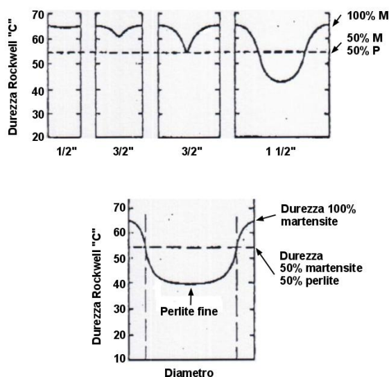
Figura 1: Curve ad U schematiche per un acciaio di composizione eutettoidica.
