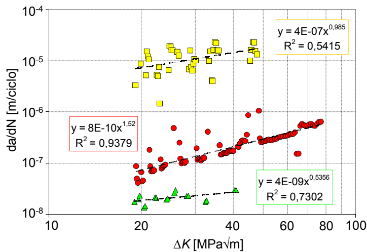
Figura 7: Risultati di prove di propagazione effettuate su campioni di acciaio 1.2738 a struttura mista costituita da martensite rinvenuta, bainite ed austenite residua modificate dal rinvenimento.
