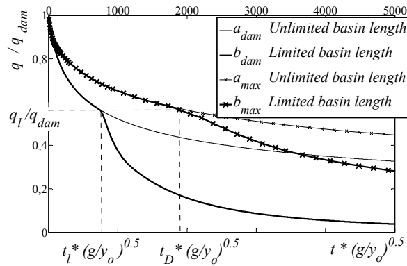
Fig. 3. Limited basin effect Influence de la longueur finie du reservoir
