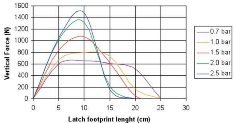
Fig. 26 - Esempio di forma del segnale in base all'impronta del veicolo. Example of signal shape based upon the vehicle print.
