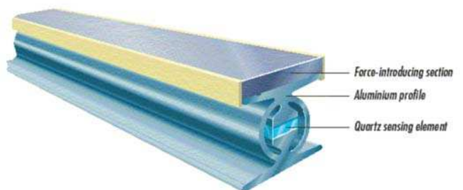
[Fonte/Source: KISTLER] Fig. 23 - Sensore al quarzo e relativa installazione. Quartz sensor and relevant installation.
