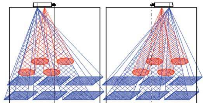
Fig. 6 - Rappresentazione dei fasci volumetrici dei sensori. Representation of the volumetric bundles of the sensors.
