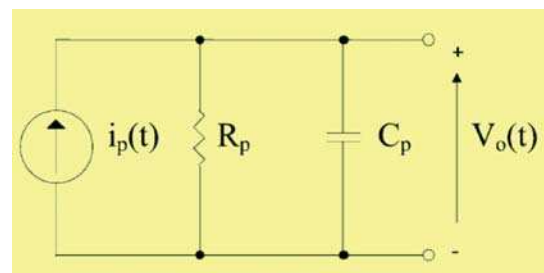
Fig. 19 - Modello elettrico elementare di un sensore piroelettrico. Elementary electrical model of a pyroelectric sensor.
