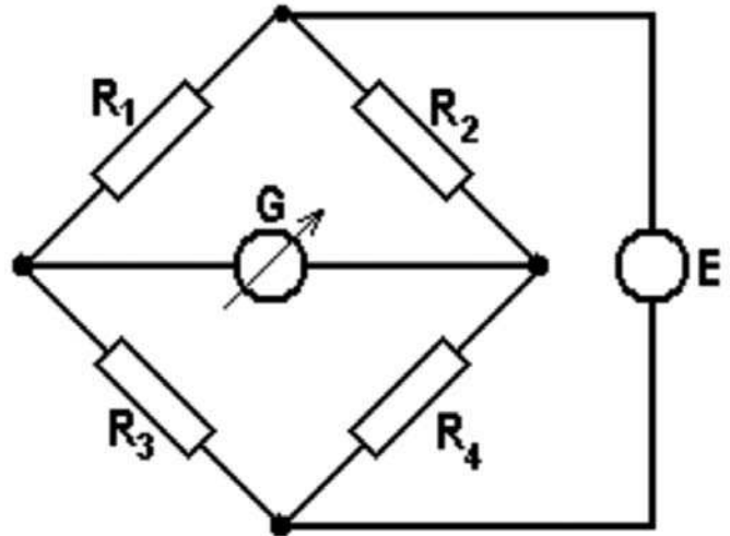
Fig. 21 - Ponte di Wheatstone. Wheatstone Bridge.
