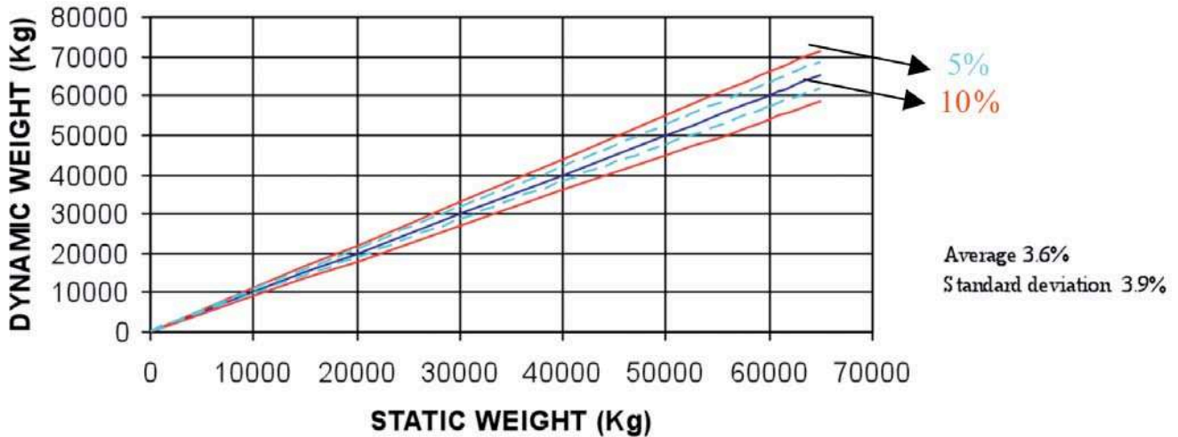
Fig. 24 - Comportamento statico e dinamico dei sensori al quarzo. Il grafico si riferisce alla pesatura di 115 veicoli. Static and dynamic behaviour of the quartz sensors. The diagram refers to the weighing of 115 vehicles.
