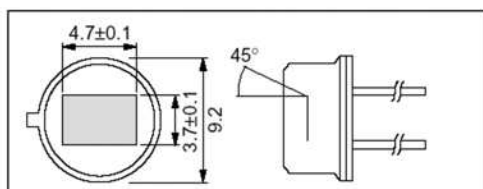
Fig. 3 - Sensore piroelettrico. Pyroelectric sensor.
