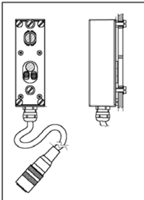
Fig. 7 - Sensore con cavo fisso. Fixed cable sensor.
