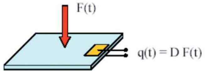
Fig. 22 – Sensore piezoelettrico. Piezoelectric sensor.
