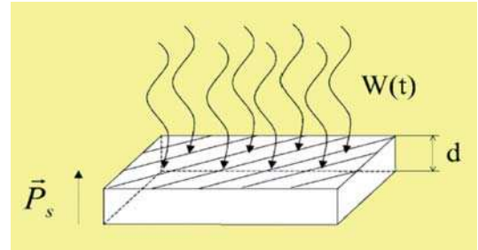
Fig. 18 - Struttura di un sensore piroelettrico piano ad elettrodi frontali. Structure of a flat pyroelectric sensor with front electrodes.
