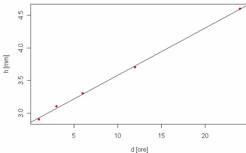
Figura A.1. Esempio di determinazione dei parametri della curva di possibilità pluviometrica a partire dai valori di altezza di precipitazione misurati sulle durate di 1, 3, 6, 12, 24 ore.
