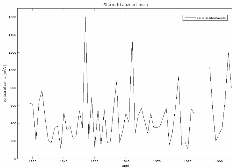
Figura 3. Serie storica di portata al colmo di riferimento definita per la Stura di Lanzo a Lanzo.
