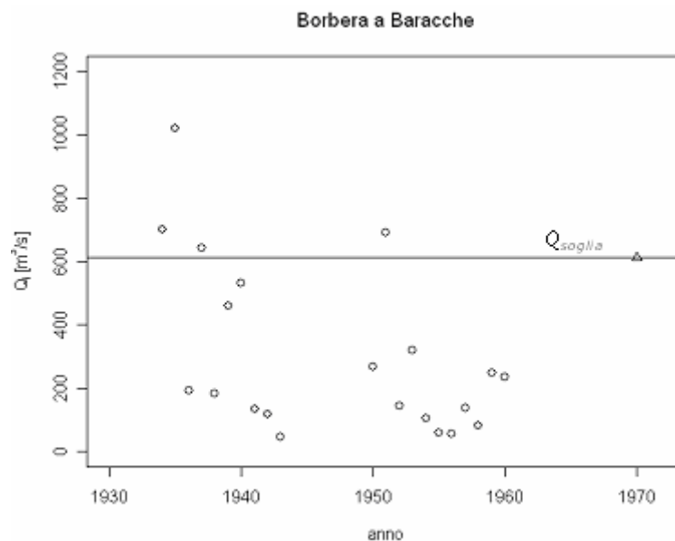
Figura B.1. Esempio di serie storica integrata con valori occasionali significativi (triangoli). Il valore della portata soglia risulta pari a 613 \text{ m}^3/\text{s} .
