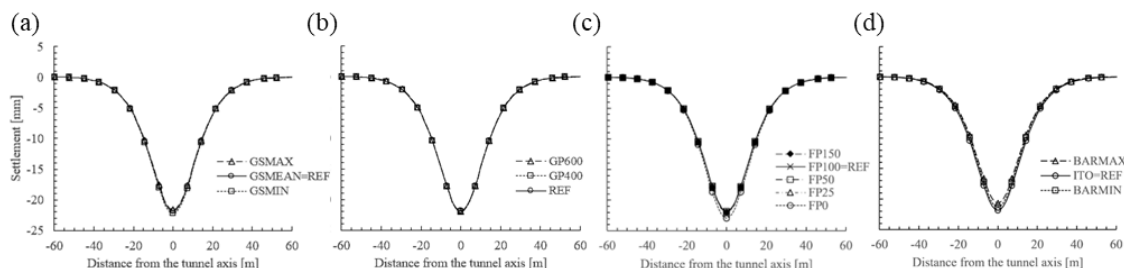
Figura 4. Profili trasversali del bacino di subsidenza al variare di: a) rigidezza della malta di riempimento; b) pressione di iniezione; c) pressione al fronte; d) parametri meccanici dei terreni.
