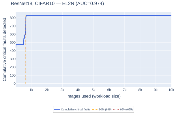
(b) EL2N
