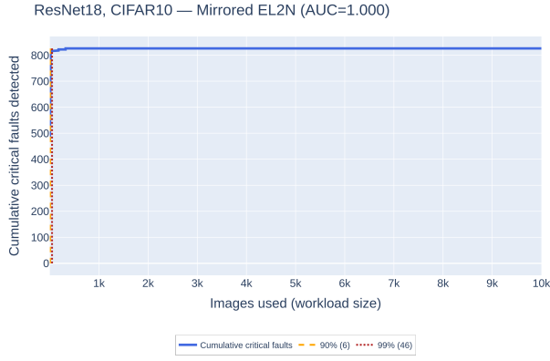
(a) MEL2N
