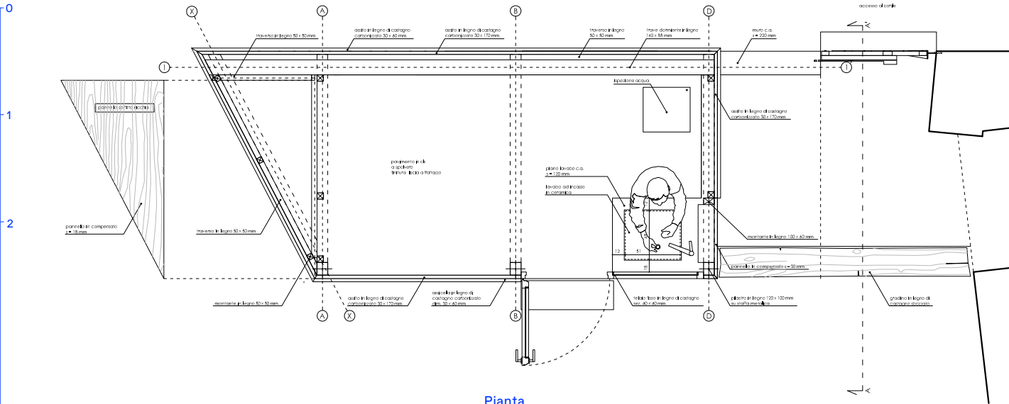
Pianta
