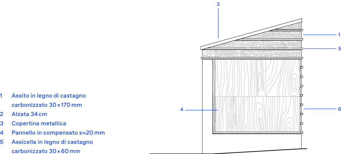
Prospetto Sud
