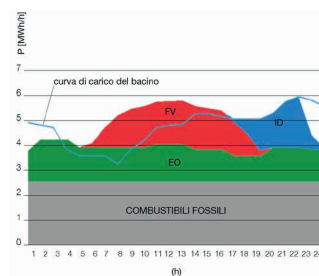
Produzione energetica giornaliera
