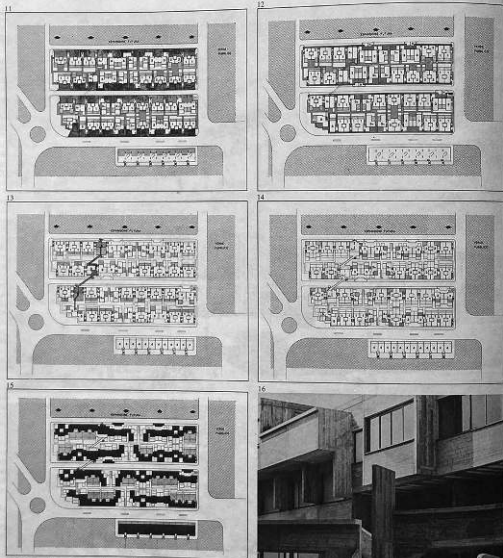
11-15 Grundriss der angelegten Etage: Erdgeschoss (11), Hochparterre (12) mit Gemeinschaftsräumen (A1-A3), erstes Obergeschoss (13), zweites Obergeschoss (14). Die Aussichts (15) plan du rez-de-chaussée: rez-de-chaussée (11), rez-de-chaussée supérieur (12), avec locaux communitaires (A1-A3), 1 er étage (13), 2 ème étage (14), plan des toitures (15). 16 Detail einer vertikalen Verbindung zur Passerelle: detail d'une liaison verticale avec la passerelle. 17 Beispiel eines Wohnungstyps: exemple d'un type de logement: 1 Kellergeschoss / sous-sol, 2 Erdgeschoss / rez-de-chaussée, 3 erstes Obergeschoss / 1 er étage, 4 zweites Obergeschoss / 2 ème étage. 18 Passerelle zum Kindergarten / passerelle conduisant à l'école collégiale.
