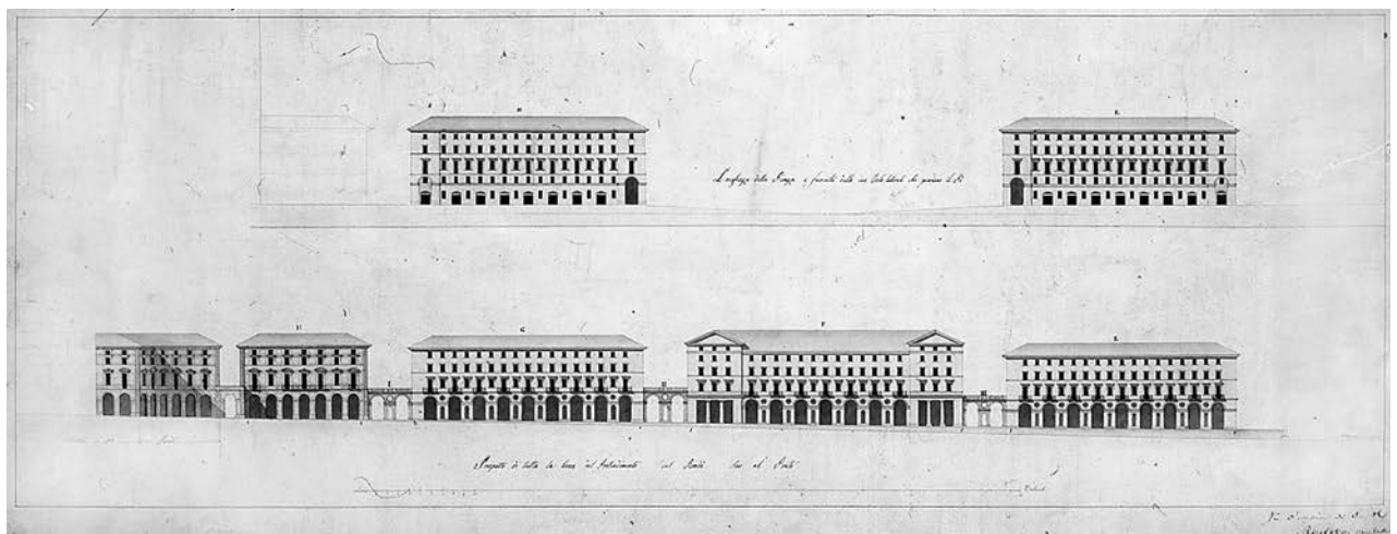
16. Giuseppe Frizzi, Disegno in pianta ed elevazione delle fabbriche con portici da farsi attorno alla grandiosa Piazza... tav. I, 1824 ca.; Torino, Archivio Storico della Città, Tipi e Disegni, 62-5-34.
