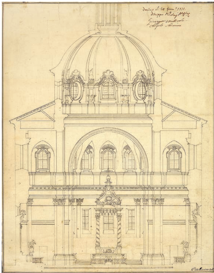
8-9. Pietro Bonvicini, Chiesa abbaziale di San Benigno Canavese, sezione e sezione parziale, 1771; Torino, collezione privata.
