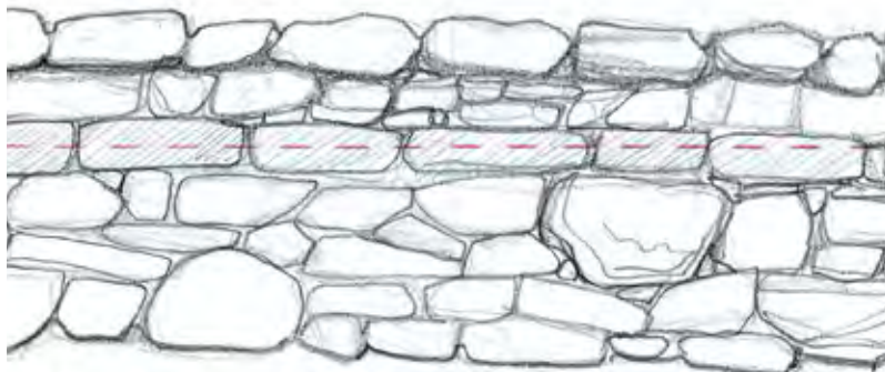
Figura 29 Corsi suborizzontali con "corso" di appianamento
