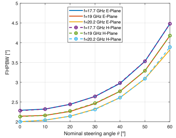
Fig. 6: FHPBW
