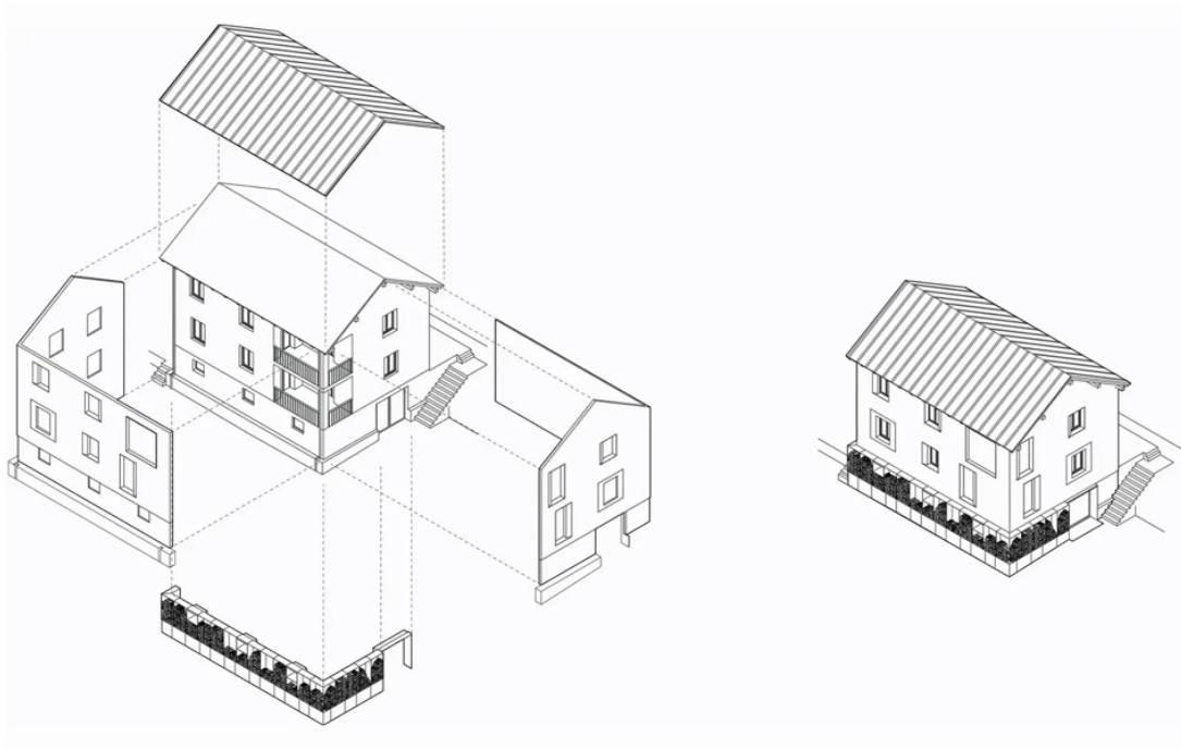
Assonometria.
