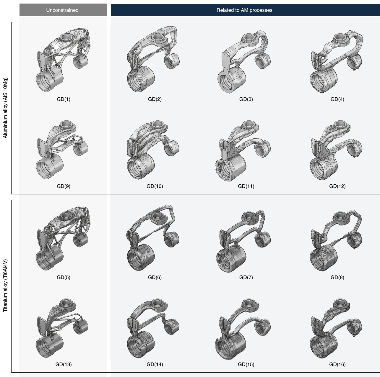
Fig. 5 GD( k ) outputs
