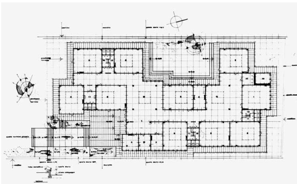
fig. 35 Claudio Conte e Leonardo Fiori, scuola elementare a 10 aule a Concesio, Brescia, 1963; pianta (da "Casabella", marzo 1964, n. 285).
