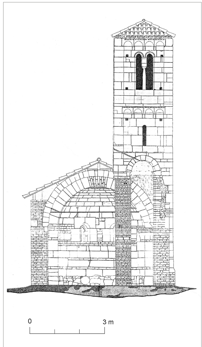
fig. 4 – Montemagno (AT), chiesa di San Vittor. Rilievo del prospetto interno absidale (arch. R. Buso 1990).
