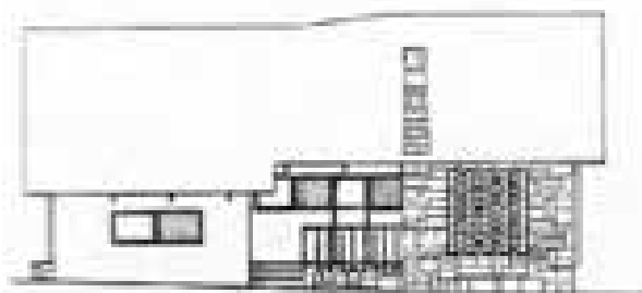
prospetto a est
