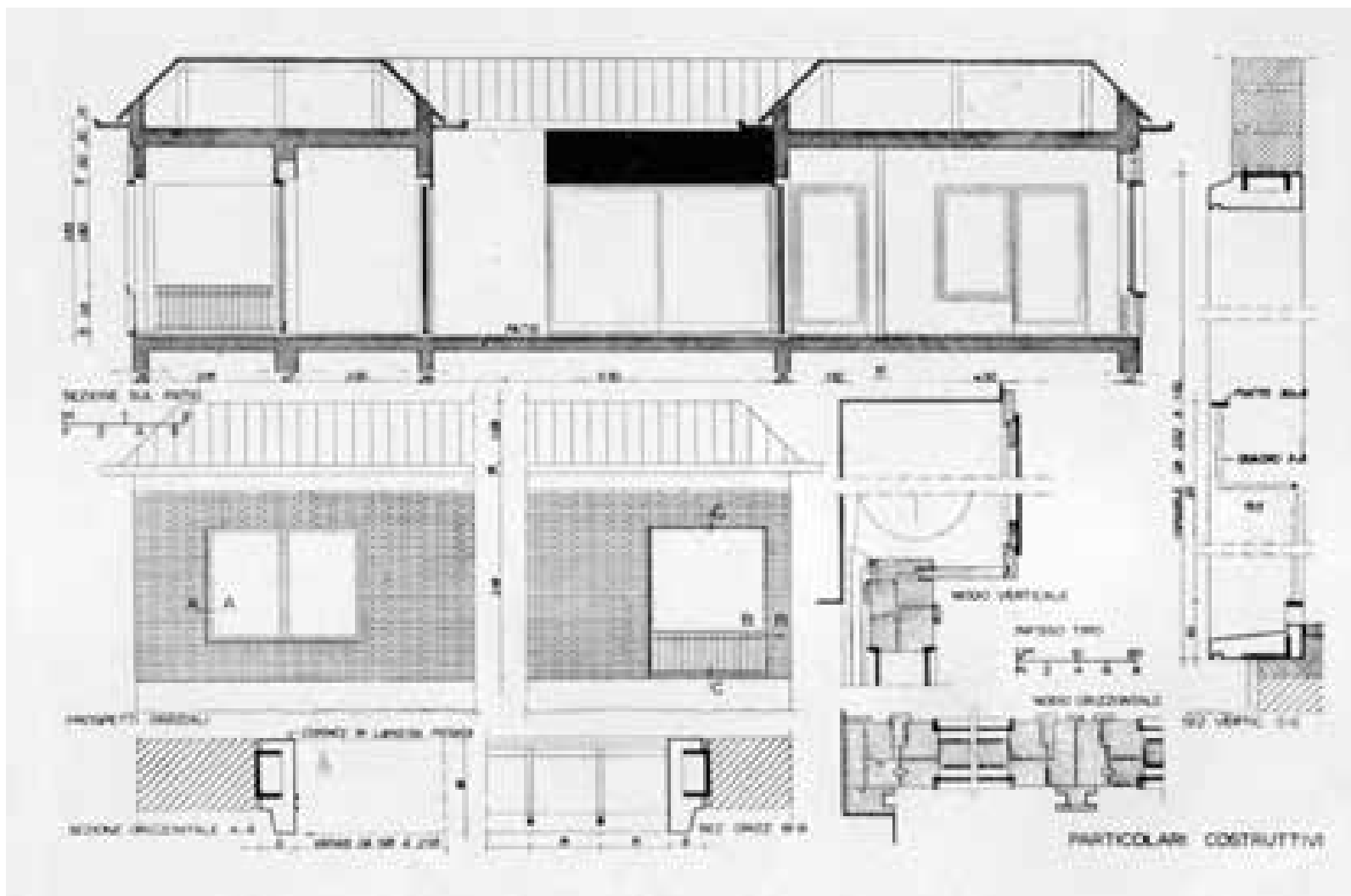
Particolari costruttivi (da Industrie e abitazioni dell'architetto Eduardo Vittoria, Villa Monterevel a Ivrea , in «L'architettura. Cronache e storia», n. 39, gennaio 1959, p. 612)
