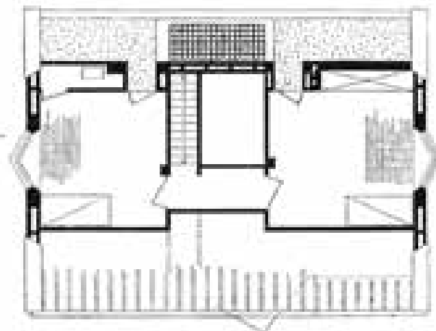
Pianta del sottotetto
