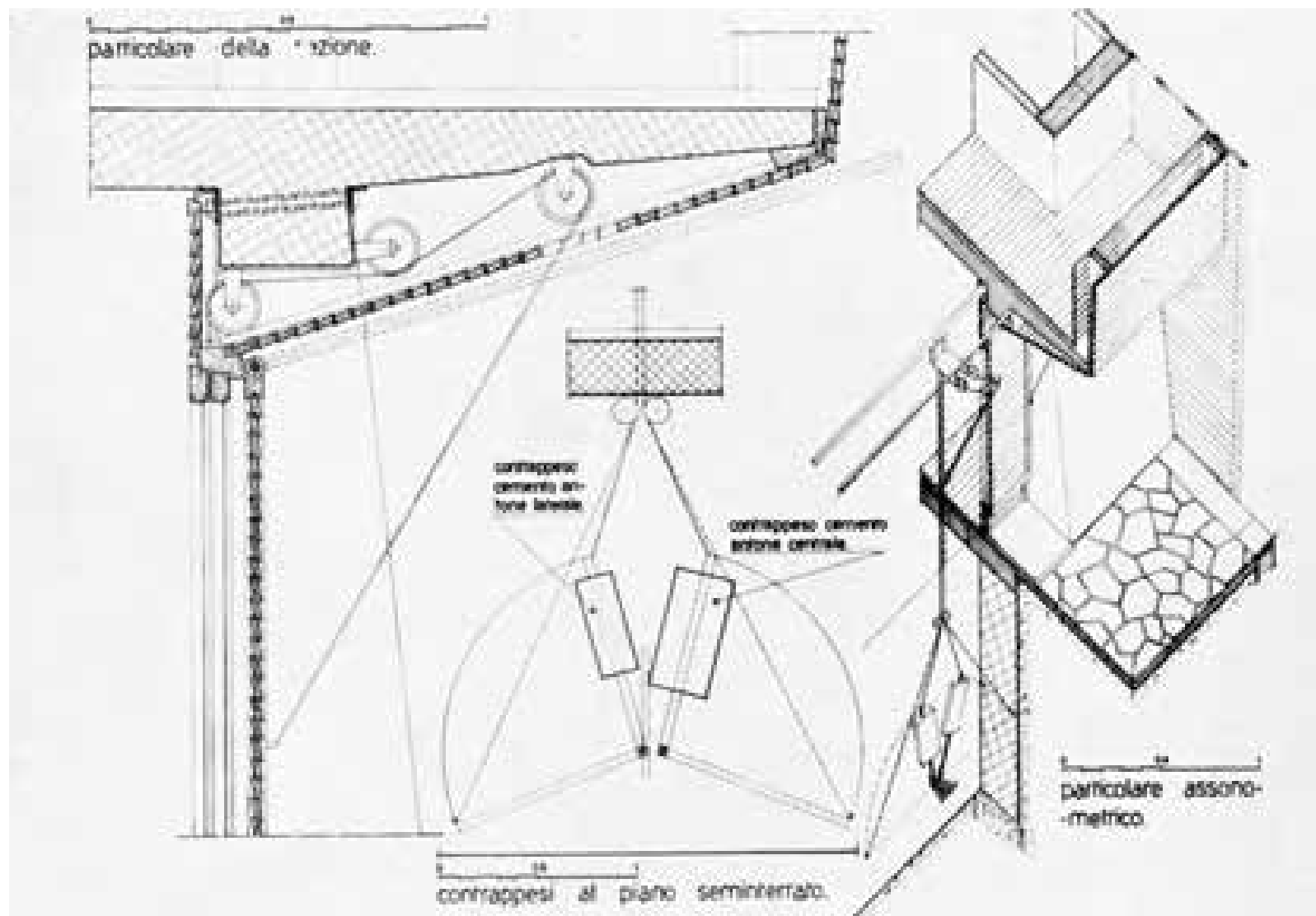
Particolare dell'apparato di manovra degli antoni per la vetrata del soggiorno (da Mario Cereghini, Costruire in montagna . Architettura e storia, Edizioni del Milione, Milano 1956, p. 194)
