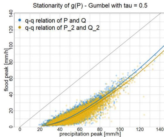
Figura 3. Confronto tra le relazioni quantile-quantile ottenute dalle distribuzioni marginali di precipitazione e portata. La correlazione tra la precipitazione e il coefficiente di deflusso è definita attraverso una copula di Gumbel ( \tau_K = 0.5 ). In azzurro le coppie di massimi annuali e la relazione q-q ottenuta con parametri di Gumbel \mu = 20 e \beta = 10 . In giallo le coppie di massimi annuali e la relazione q-q ottenute incrementando del 10% i parametri della distribuzione.
