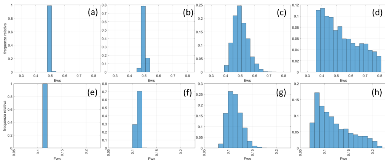
Figura 1. Frequenza relativa dell'efficienza nel risparmio idrico a confronto tra gli edifici DH (a-d) e MRB (e-h) localizzati a Crotone e dotati di una cisterna di 9 m 3 e 6.6 m 3 , rispettivamente: (a) ed (e), variabilità giornaliera; (b) ed (f), periodi a domanda costante di circa 8 mesi (0,7 anni); (c) e (g), periodi di 14 anni; (d) ed (h), un unico periodo di 70 anni.
