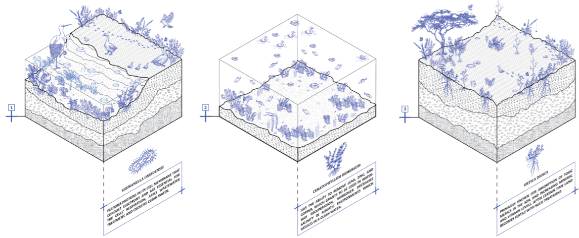
Şekil. Copperbelt katalizörleri
