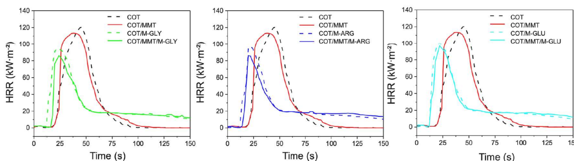
Fig. 14. HRR curves of COT, COT/MMT, COT/PAAs and COT/MMT/PAAs. Add-ons: 2 % MMT in COT/MMT; 2 % MMT and 14 % PAA in COT/MMT/PAA samples.
