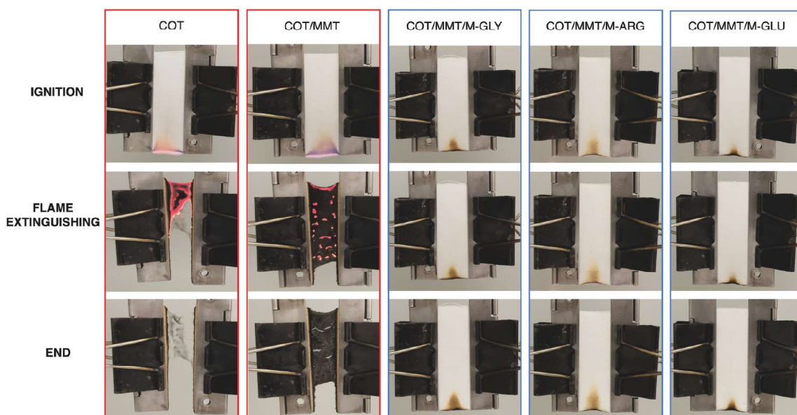
Fig. 13. Snapshots of VFSTs carried out on COT, COT/MMT and COT/MMT/PAA samples. Add-ons: 2 % MMT in COT/MMT; 2 % MMT and 14 % PAA in COT/MMT/PAA samples.
