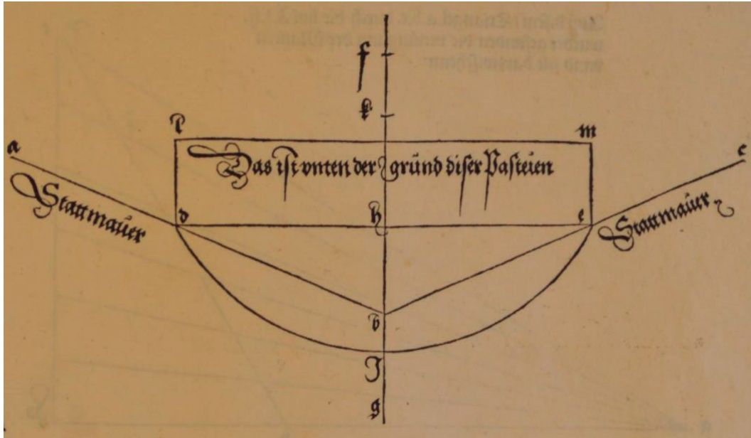
Albrecht Dürer (1527, f. 3r), Pianta del bastione .
