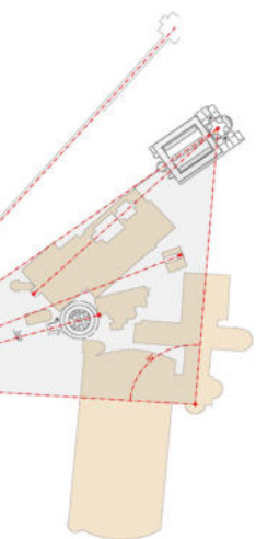
Prima azione. Tracciamento dell'asse policentrico passante per la Rotonda del Parco e centrato sul cosiddetto Palatium Invernale, del Ninfeo Stadio, dell'Edificio con tre Esedre e del Pecile. Prima grande trilaterazione.
