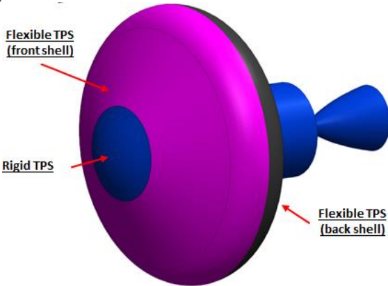
Fig. 17: TPS layout.
