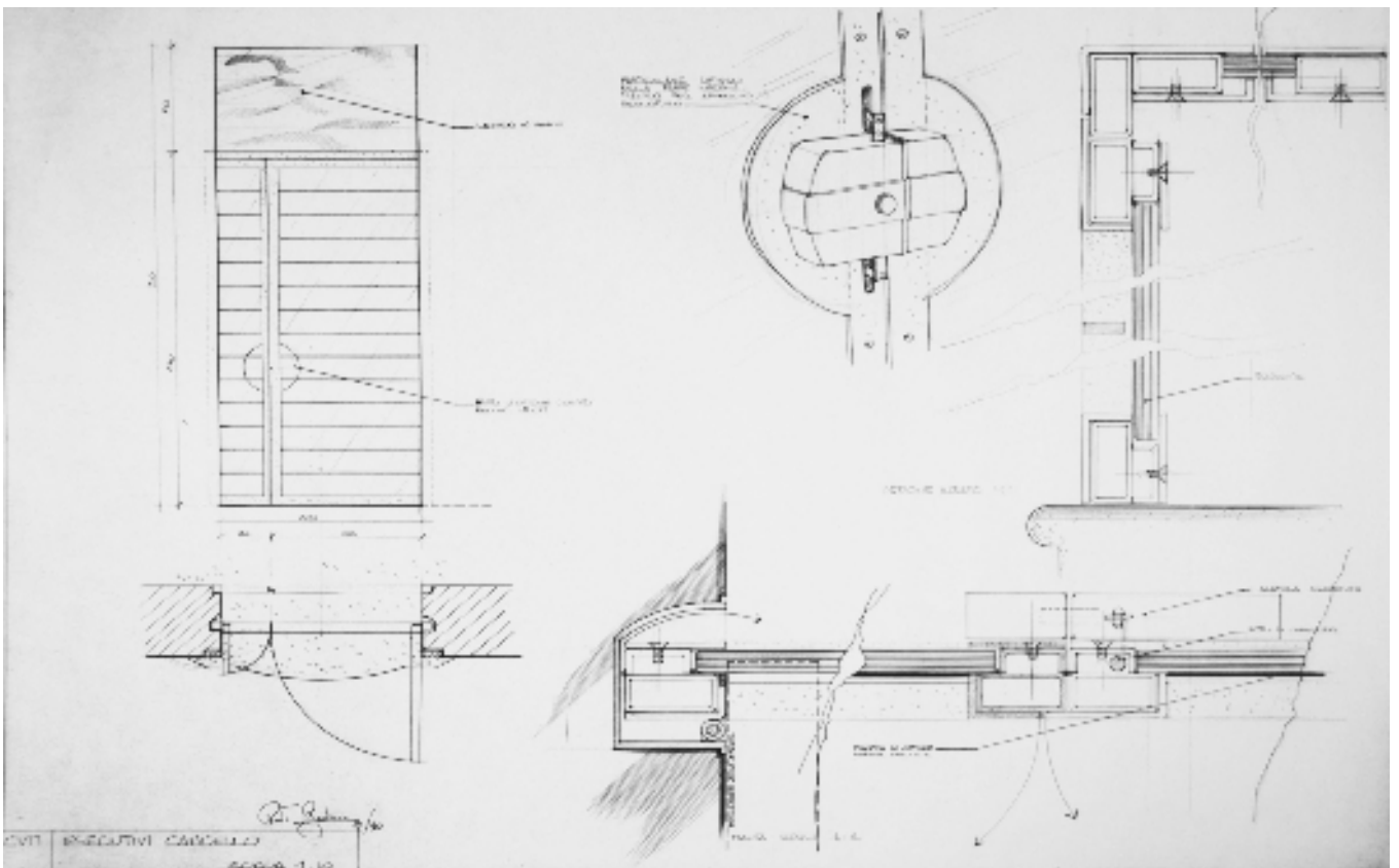
Progetto 25. 1989–90. Appartamento V. Bologna. Con Roberto Gresleri.
