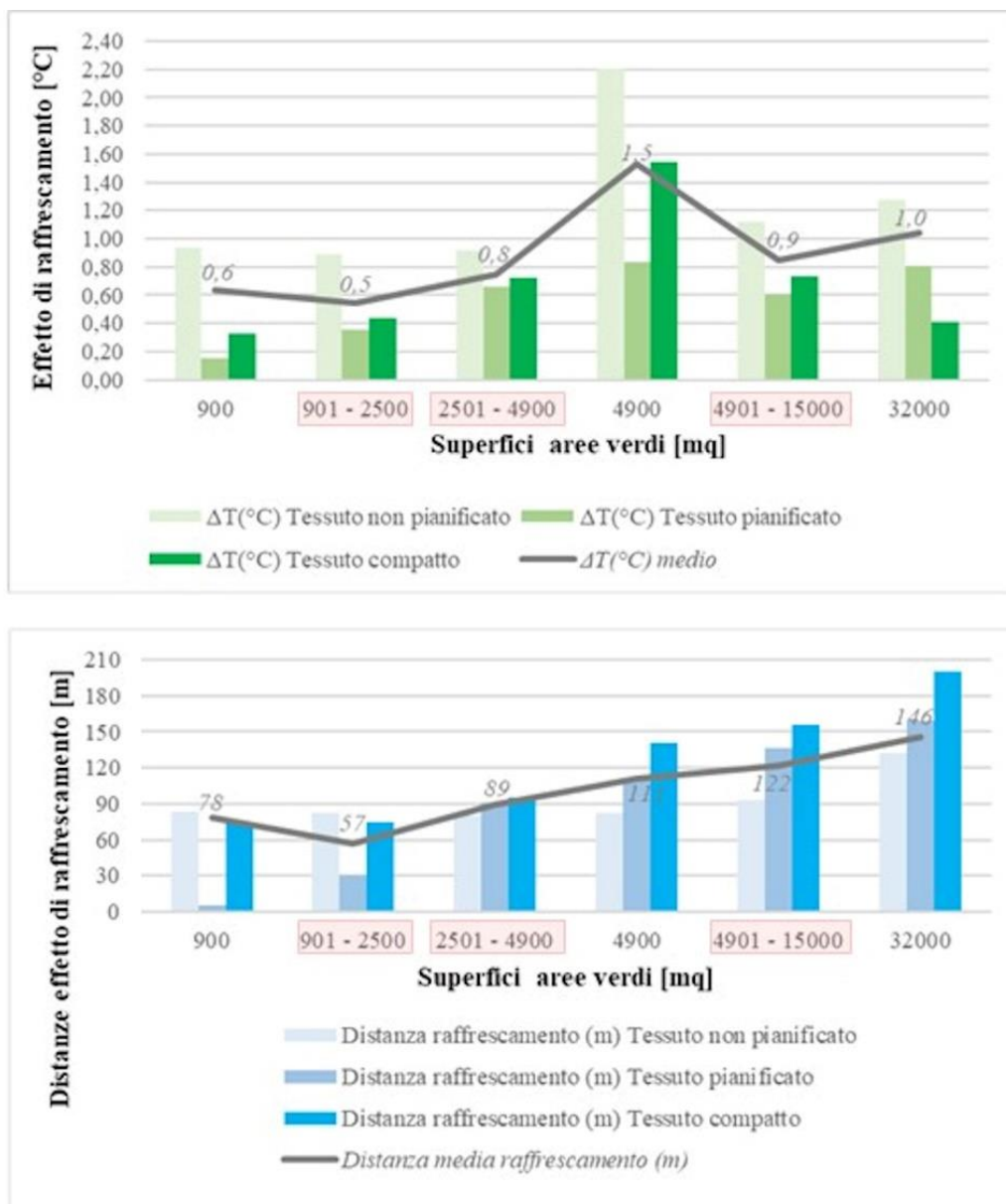
Figura 1 | Effetti di raffrescamento di riferimento e relativi a Cercola (in rosso).
