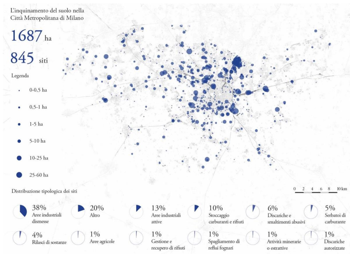
Figura 2 | Distribuzione delle aree contaminate e potenzialmente contaminate puntualmente nel territorio metropolitano milanese. Fonte: elaborazione di Lucia Ludovici su dati estrapolati dal Database AGISCO, Arpa Lombardia, aggiornato ad aprile 2021 e dai DBT del Geoportale Regione Lombardia e Geoportale Regione Piemonte.
