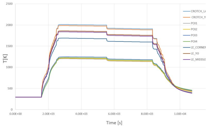
Fig. 8. Air intake POI thermal behavior
