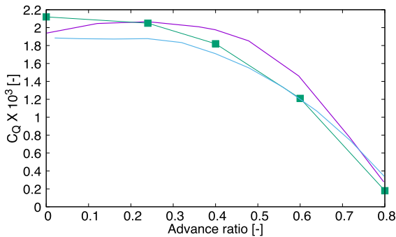
Fig. 20. Torque coefficient.
