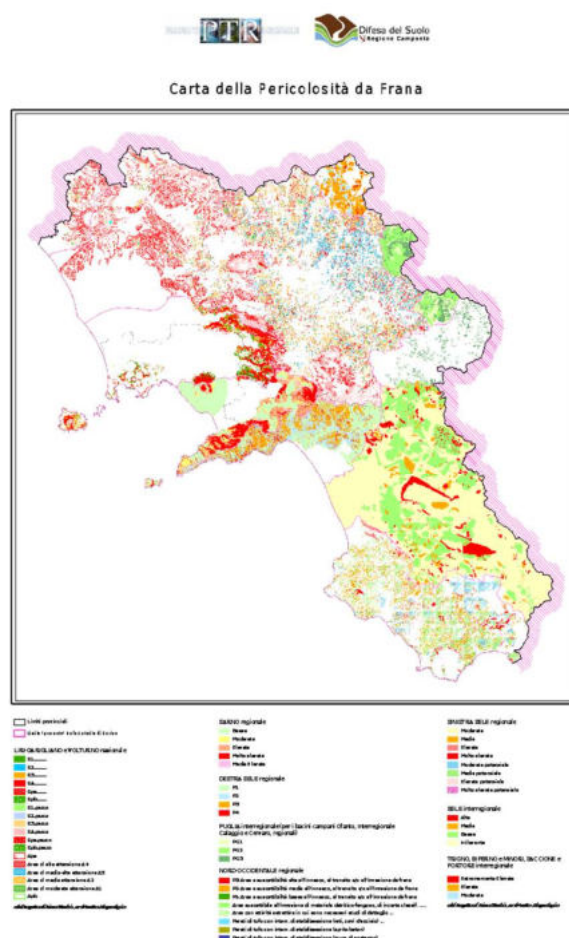
Fig. 2 - Pericolosità da frana
