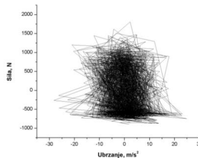
Slika 6 - Zavisnost sile od relativnog ubrzanja za amortizer A i za efektivnu amplitudu od 10 mm
