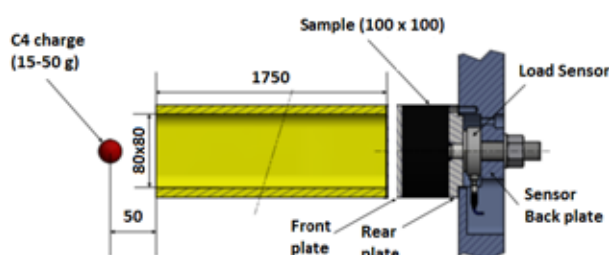
Fig.1 EDST schematic
