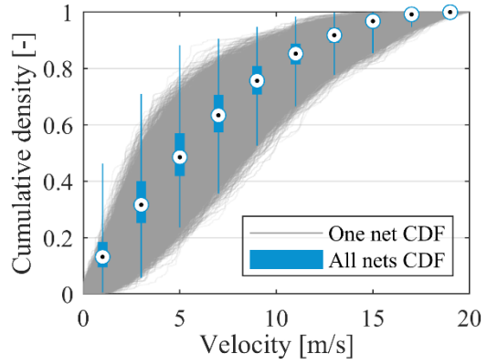
(D) Statistical distributions of gas flow velocities in pipes
