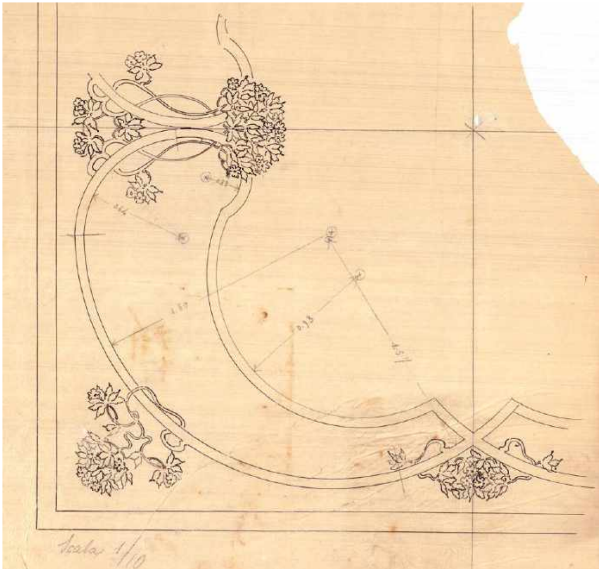
Fig. 17. Carlo Musso, soffitto in stile Moderno , inchiostro su velina, scala 1:10, s.d. Torino, Politecnico di Torino, DIST – LSBC, Fondo Musso Clemente , MC.266.
