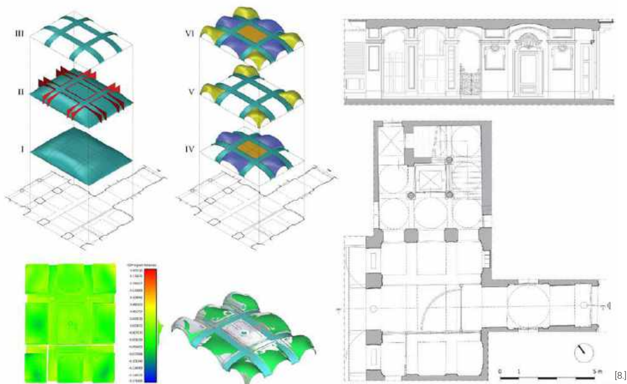
Fig. 7. Palazzo Capris di Cigliè , Torino. Pianta e sezione in scala 1:50 dell'atrio e rappresentazione, in esploso assonometrico, del modello interpretativo del sistema voltato [disegni e modelli digitali a cura di Fabrizio Natta].
