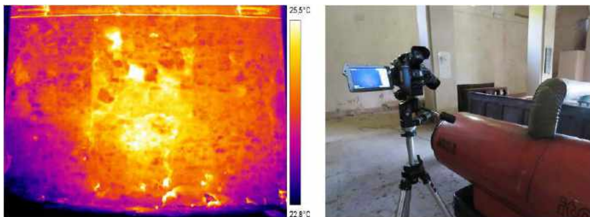
Fig. 4. Termogramma IR (sinistra) e postazione di rilievo (destra) [elaborazione a cura degli autori].
