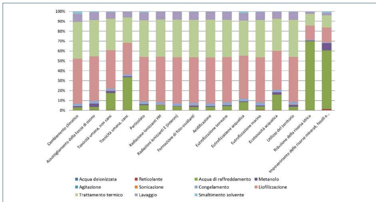
Figura 3. Contributi relativi delle voci di processo all'impatto totale della produzione di nanopugne di cellulosa in scala laboratorio
