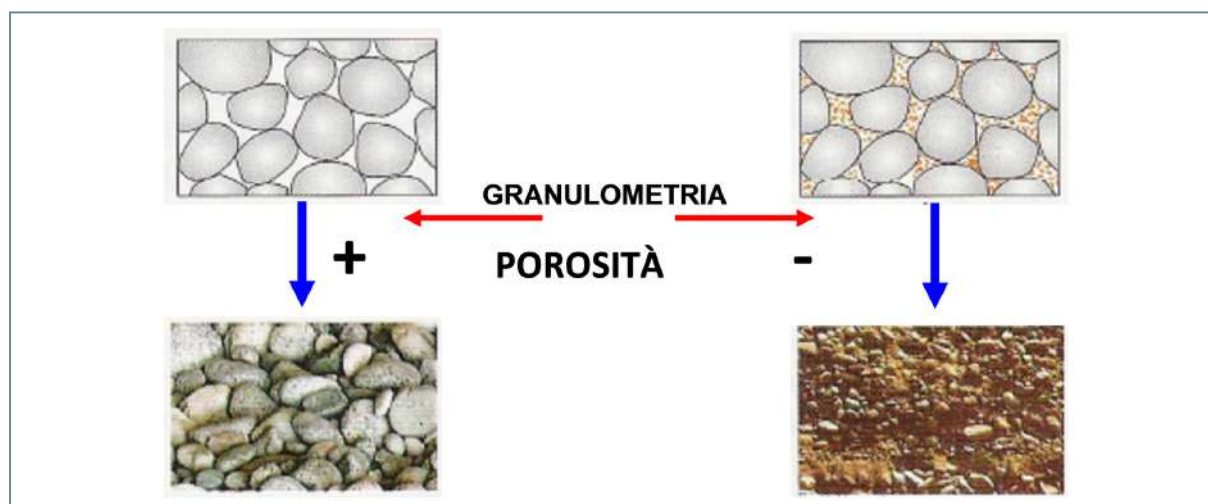
Figura 9. Rapporti tra granulometria delle rocce incoerenti e la loro Porosità
