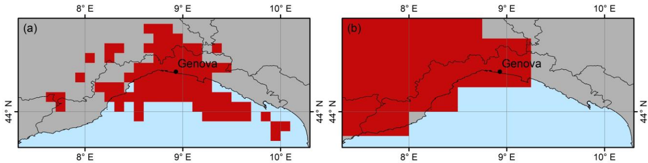
Figura 3. Rappresentazione spaziale delle allerte prodotte da ERDS. Figura 3a: aree allertate durante il periodo 23/11/2019 - 25/11/2019 (prima di tali date non sono state fornite allerte) utilizzando il dato GPM come input. Figura 3b: allerte prodotte a partire dal dato GFS nel periodo 20/11/2019 - 24/11/2019.
