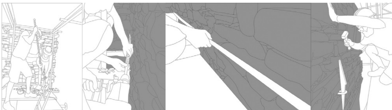
Fig. 3. Da sinistra: preparazione del trapano carotatore; foraggio del muro tramite trapano carotatore; inserimento dei tiranti nelle scanalature; inserimento del capochiave nell'occhiello del tirante © 2018, Rielaborazione degli autori.
